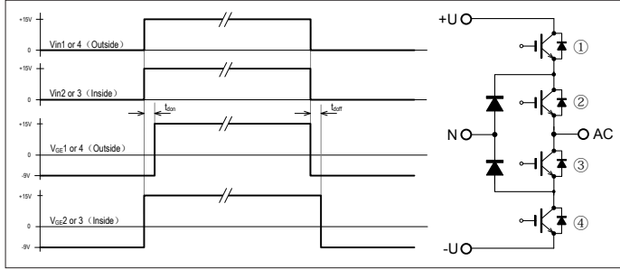
图 2.2.1, 时序管理波形示意图
