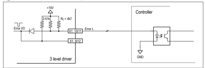
图 2.3.3 故障输出驱动光耦的接口示意图
