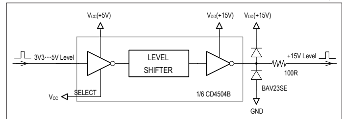
图 2.1, CD4504B 构成的电平转换电路
