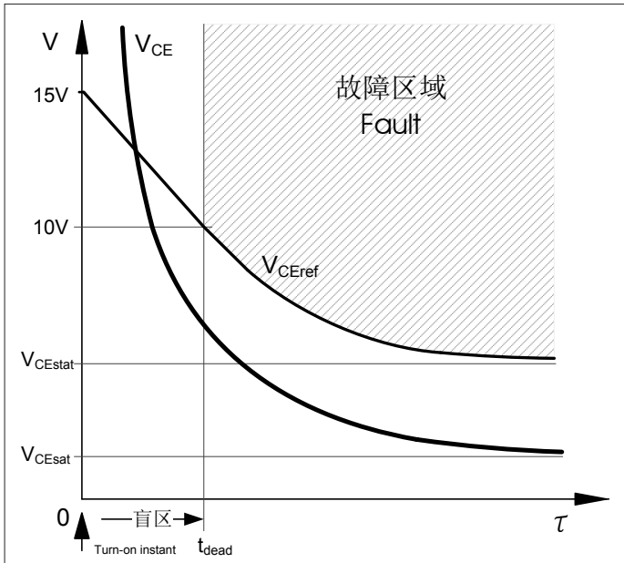
图 2.14 V CEsat 电压监控曲线 V CEref 及 IGBT 导通瞬间的 V CE 电压波形示意图
