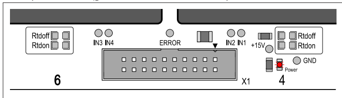
图 2.2.2, 时序时间设置电阻 R_{tdON} 及 R_{tdOFF} 焊盘位置示意图
