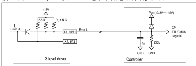
图 2.3.2 控制侧低于 15V 电平的故障输出接口示意图
