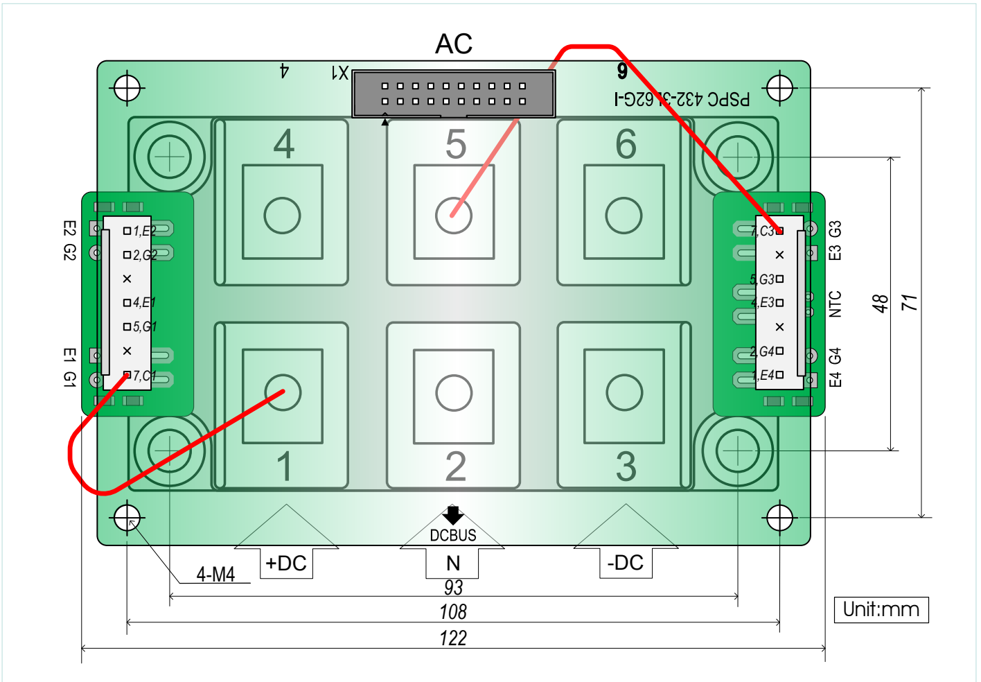
装配示意图
