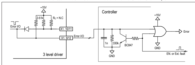
图 2.3.1 故障输出带使能控制接口示意图
